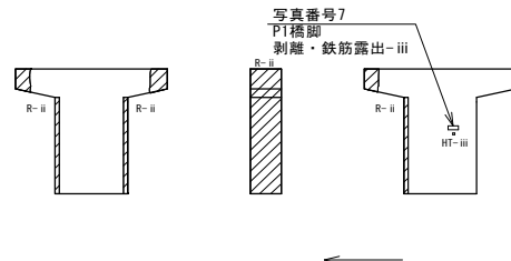
P 1 橋脚
