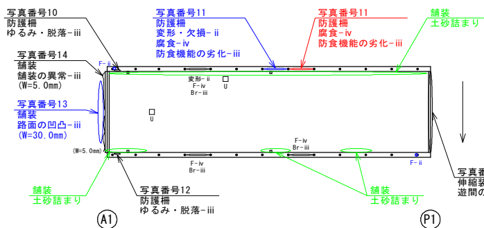
A 1 橋台
