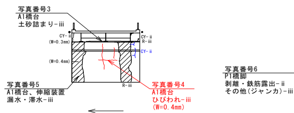
A 1 橋台
